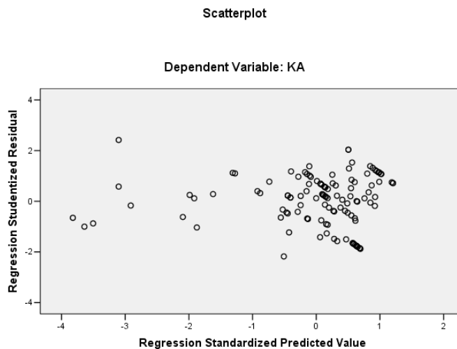
Gambar 2. Uji Heteroskedastisitas
