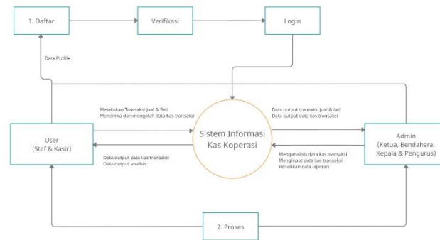
Gambar 3 Gambar DFD Level 1
