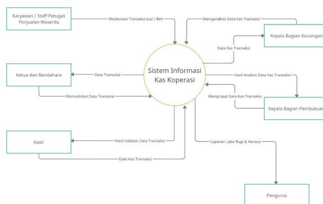
Gambar 1 Gambar Konteks Diagram
