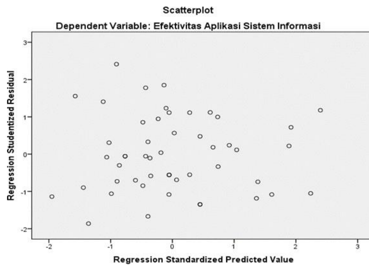
Gambar 4 Uji Heteroskedastisitas
